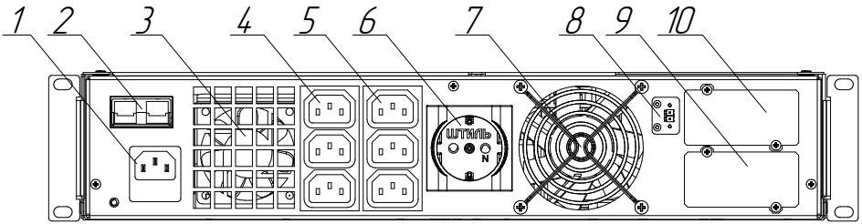
Рисунок 8. Компоненты задней панели ИБП Штиль STR1101LD
