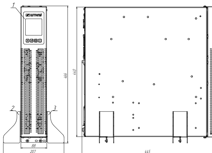
Рисунок 6б. Габаритные размеры и компоненты ИБП Штиль STR1102L, STR1103L и STR1103TL (вертикальная напольная установка)
