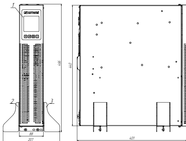
Рисунок 4б. Габаритные размеры и компоненты ИБП Штиль STR1101L, STR1101SL и STR1101LD (вертикальная напольная установка)
